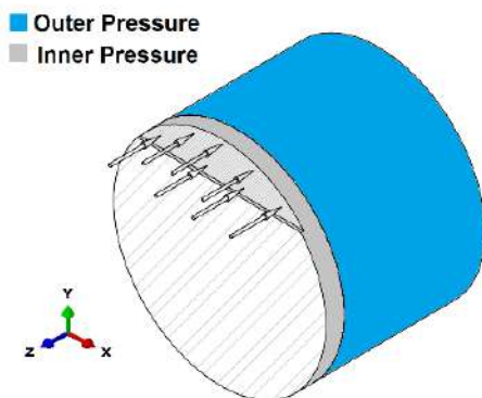
Figura 9: Esquema de la condición de carga de la probeta en ensayo de fractura con confinamiento.
