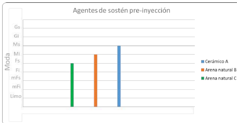
Figura 5. Este gráfico muestra la moda (tamaño de grano que corresponde a la mayor frecuencia) de cada muestra pre-inyección.
