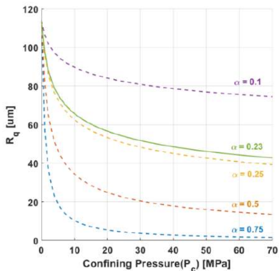
Figura 21: Estimación de R_q a partir del modelo basado en P_c (ec. 1) para diferentes exponentes \alpha . Suponemos R_q|_{(P_c=0)} = 114 constante para todo valor de \alpha . La línea verde sólida corresponde al modelo ajustado para nuestras pruebas.
