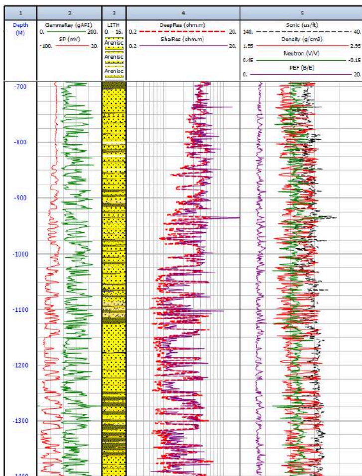
Figura 4: Perfil tipo en el área de estudio. Track 1, profundidad en metros referidos al nivel del mar. Track 2, Potencial espontáneo SP (rojo) y rayos gamma GR (verde). Track 3, litología interpretada del control geológico. Track 4, resistividad profunda (rojo punteado) y somera (morada). Track 5, densidad (rojo), neutrón (verde), factor fotoeléctrico PEF (morado) y sónico (negro punteado).
