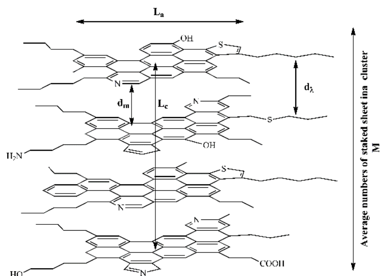
Figura 2. Vista en sección transversal de la estructura de un clúster de asfaltenos con los principales parámetros cristalinos.
