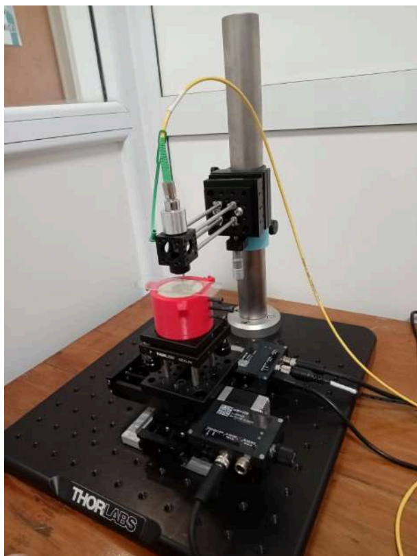
Figura 14: Interferómetro.
