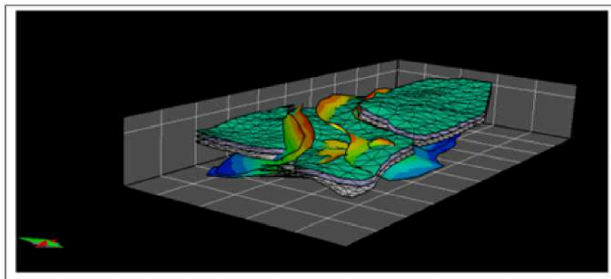
Figura 6: Modelo estructural 3D de la zona de Puesto Touquet. Las superficies de colores azul a rojo representan fallas y las superficies grilladas representan los topes del basamento, la Fm. Molles y el Mb Cutral-Co.
