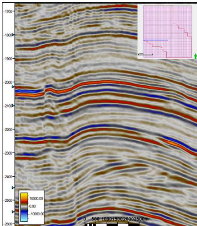
Figura 14. Corte sísmico de PSDM procesada a partir de registraci3n con nodos y barridos DSS, coincidente con corte sísmico de la Figura 13.
