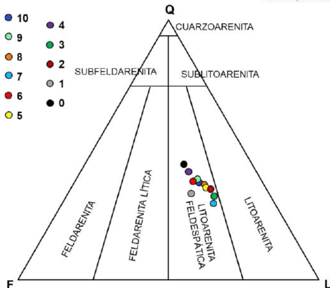
Figura 6: Composición litológica y diagrama de QFL (Folk et al. [15]). Los puntos de colores representan las muestras de roca de la Formación Centenario. Nótese que todas caen
