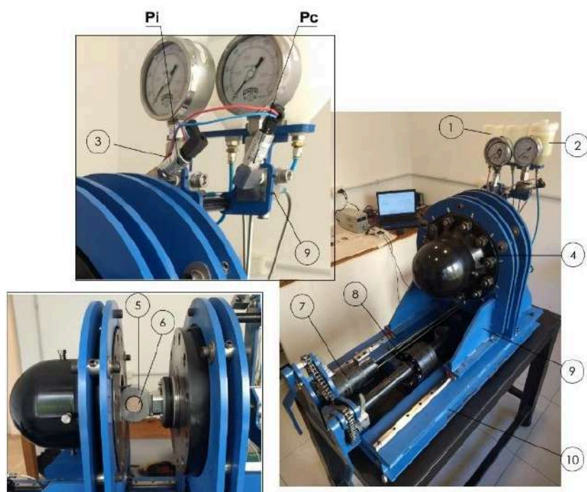
Figura 1: Esquema de RTT. Partes principales: (1-2) Depósitos de fluidos interiores y exteriores, (3-9) Colectores y transductor de presión P_i y P_c , (4) Cámara externa ( P_c ), (5) Cámara de presión interior, (6) Muestra de roca, (7-8) Intensificador de presión para fluidos interiores y exteriores, (10) Base fija, (11) Base Móvil.
